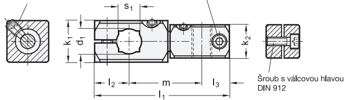
Upínací sada GN 511
